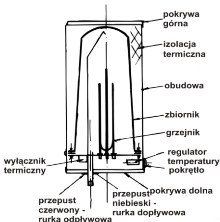
Rys. 2 Budowa ogrzewacza
