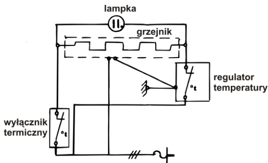
Rys. 3 Schemat elektryczny
